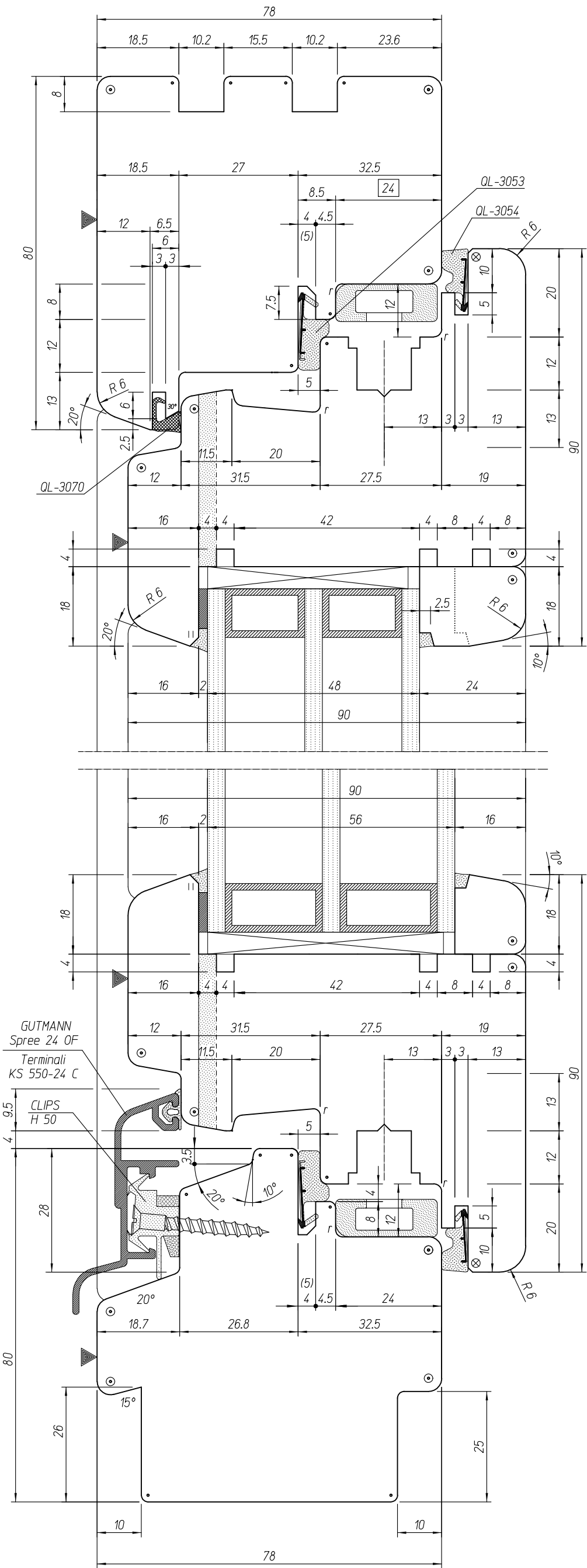
SEZIONE VERTICALE
