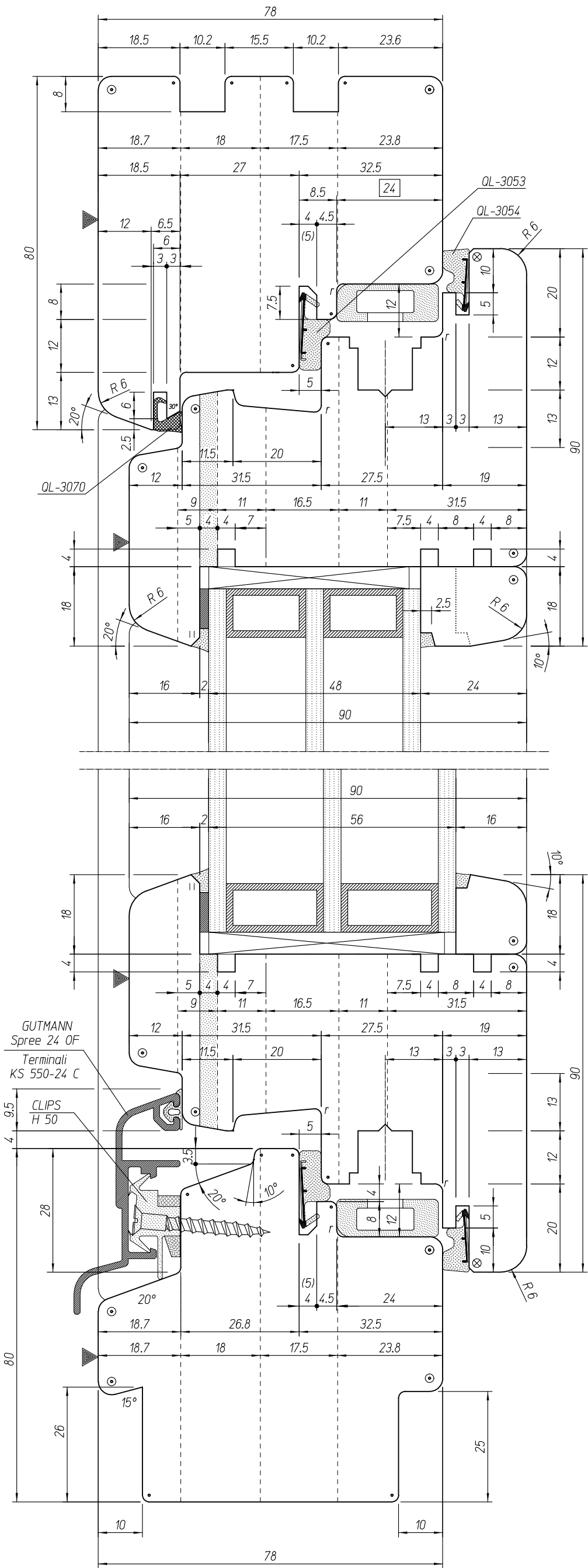
SEZIONE VERTICALE
